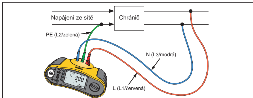
Obrázek 18. Schéma zapojení při testování chráničů na IT síti.
