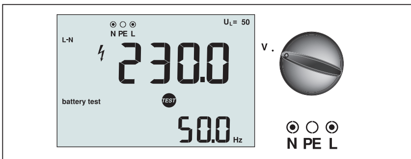
Obrázek 8. Zobrazení napětí/Nastavení přepínače a vstupních zdířek apx002f.eps
