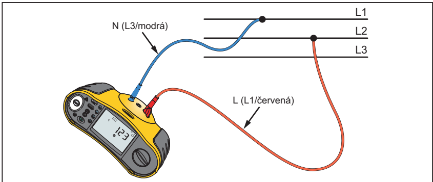
Obrázek 15. Měření na 3-fázové síti
