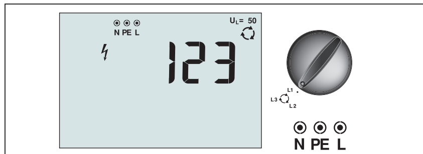
Obrázek 21. Zobrazení sledu fází/Nastavení přepínače a vstupních zdířek
