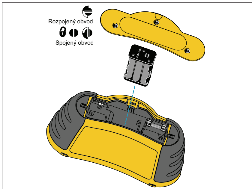
Obrázek 24. Výměna baterií
