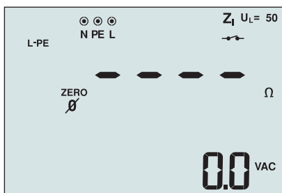
Obrázek 12. Displej po vynulování
