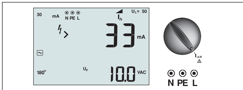
Obrázek 17. Vypínací proud chrániče/Nastavení přepínače a vstupních zdírek
