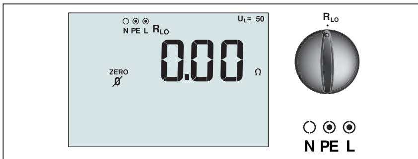
Obrázek 10. Zobrazení nuly spojitosti/Nastavení přepínače a vstupních zdířek
