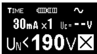
Obr. 3.11 Příklad nastavení pro měření vypínacího času
