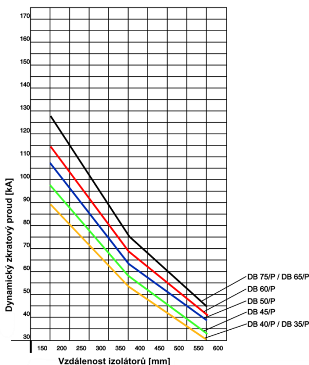
Graf zkratové odolnosti č. 3
