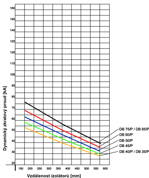
Graf zkratové odolnosti č. 4
