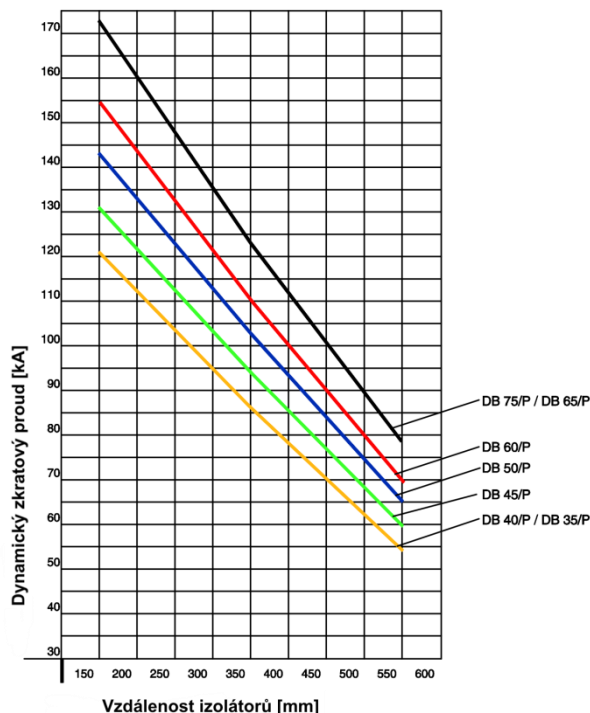
Graf zkratové odolnosti č. 1
