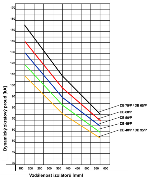
Graf zkratové odolnosti č. 2
