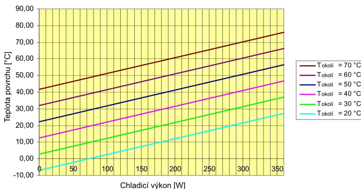
Graf chladicího výkonu GN-316-C
