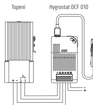
Příklad zapojení
