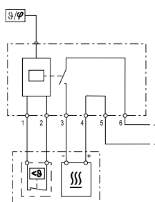
Schéma připojení
