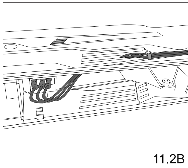
11.B Meldeschalter - Kabelverlegung außen Pilot switch - cable routing outside
