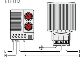
Příklad zapojení
