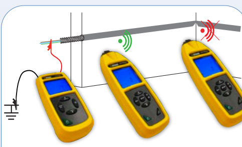
Detekujte zúženou (nebo ucpanou) část nekovové trubky (vyžaduje dočasné vložení vodiče)
