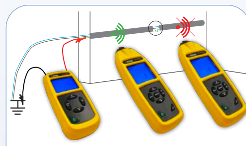
Lokalizujte přerušení vedení
