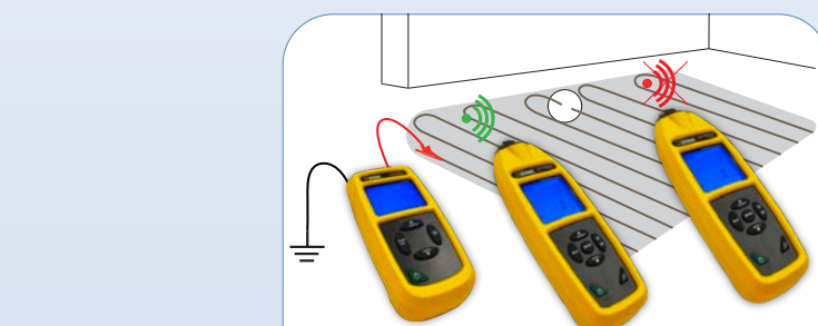
Detekce závad v podlahovém vytápění (nestíněný)
