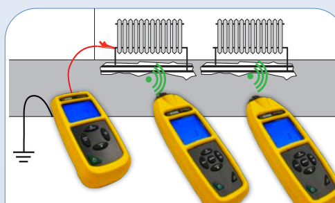
Detekce kovového topného potrubí
